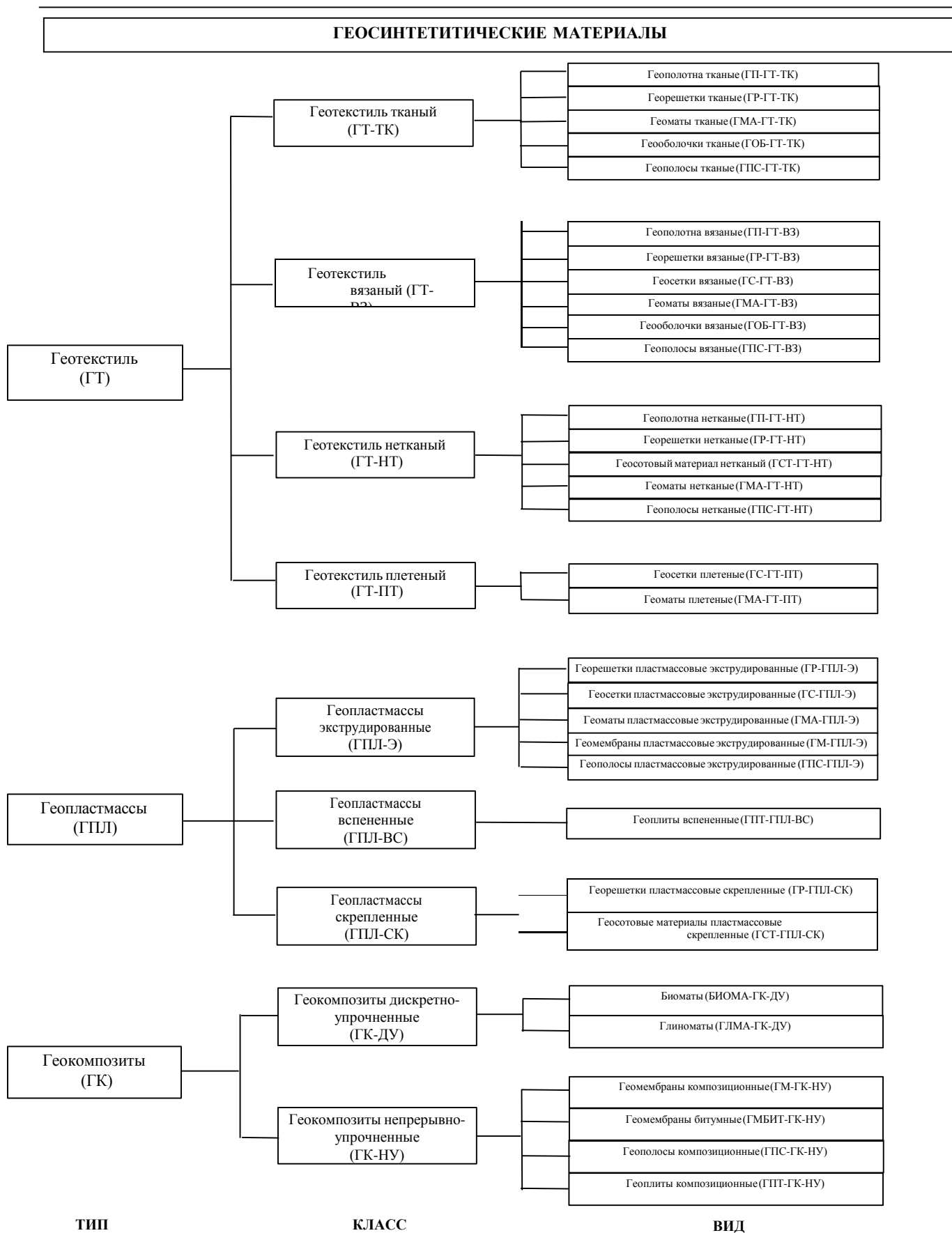
Рисунок 1 – Общая классификация геосинтетических материалов
