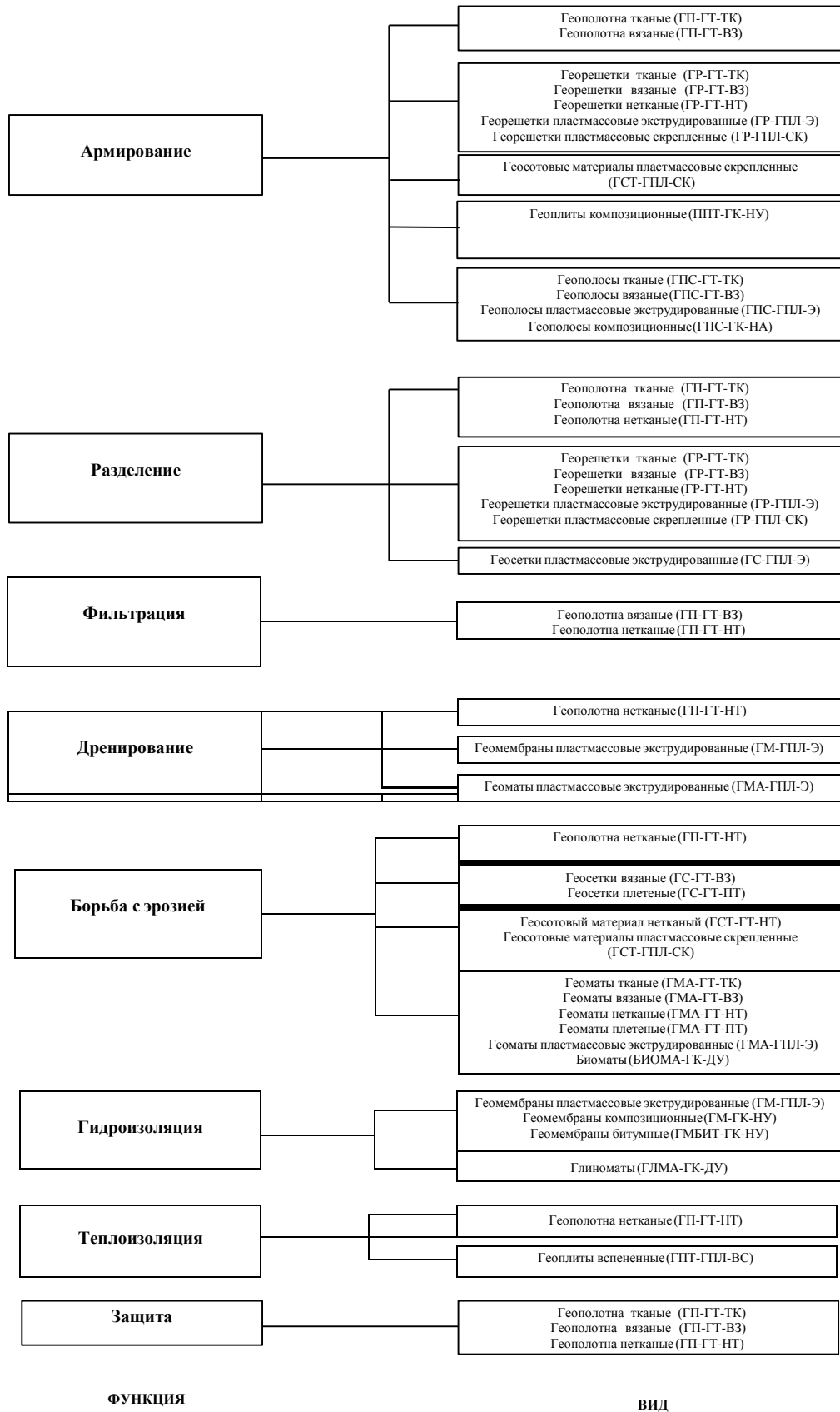
Рисунок 2 – Классификация геосинтетических материалов по функциям применительно к дорожному строительству
